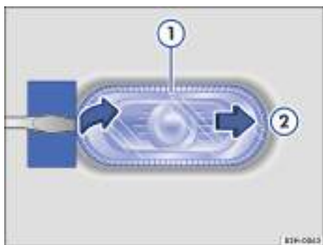
Fig. 153 En el lateral del vehículo: desmontar el intermitente lateral.
