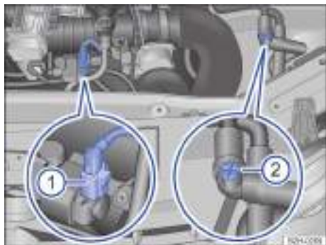
Fig. 181 En el vano motor: conector y válvula de purga manual.
