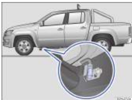
Fig. 134 En los bajos del vehículo, en el larguero: tornillo de desagüe de filtro del gasóleo (en función del equipamiento).
