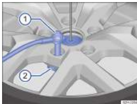
Fig. 201 Rueda de repuesto o de emergencia: colocar el tornillo de seguridad.
