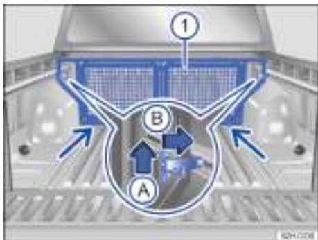
Fig. 128 En la superficie de carga: montar el elemento divisorio.
