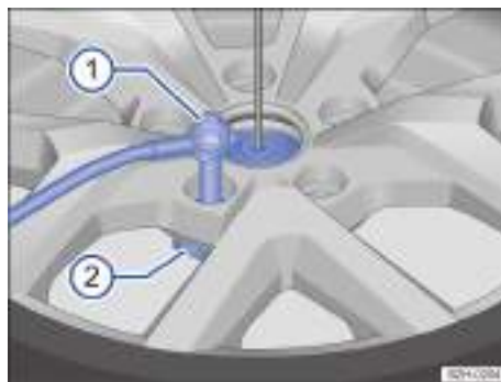
Fig. 198 Rueda de repuesto o de emergencia: soltar el tornillo de seguridad.
