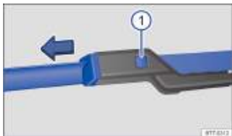
Fig. 142 En el parabrisas: cambio de las escobillas limpiacristales del parabrisas.
