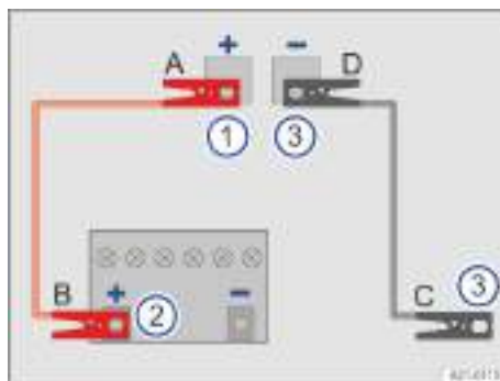
Fig. 165 Esquema para la conexión de los cables de arranque.
