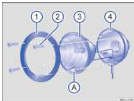
Fig. 157 Faro adicional en el techo del vehículo: desmontar el cristal.
